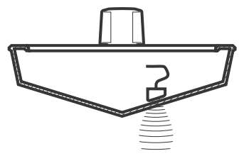
Installation du transducteur angulaire
