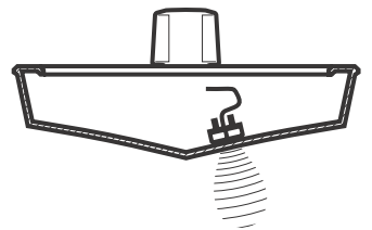
Installation du transducteur angulaire
